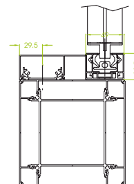
Profilé d'intégration
