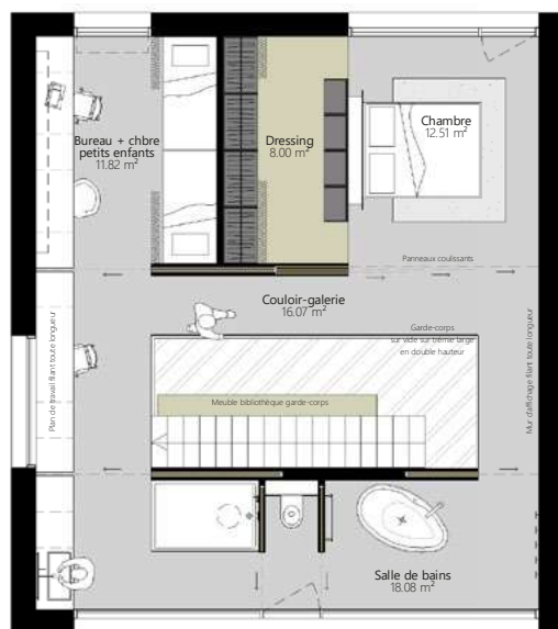
Plan étage
